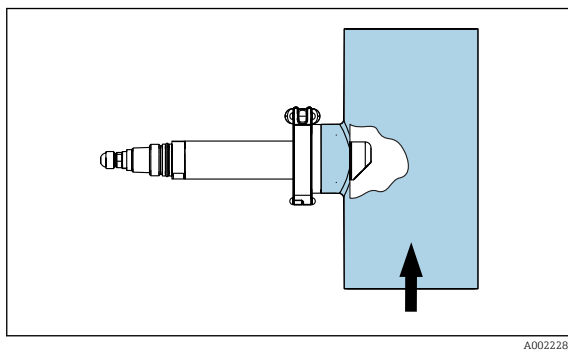
18 Монтаж с проточной арматурой CUA262
