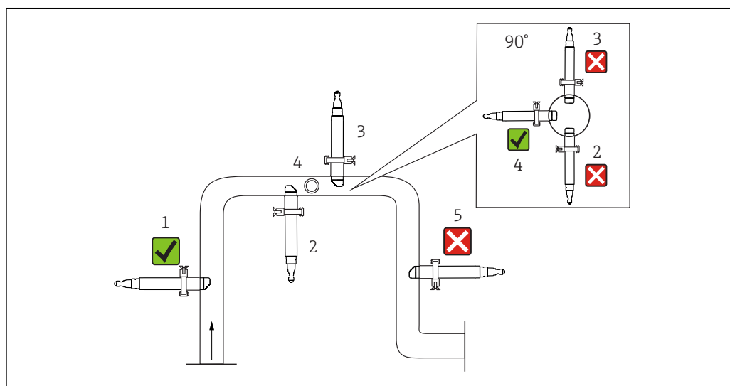
11 Допустимые и неприемлемые варианты ориентации в трубах
