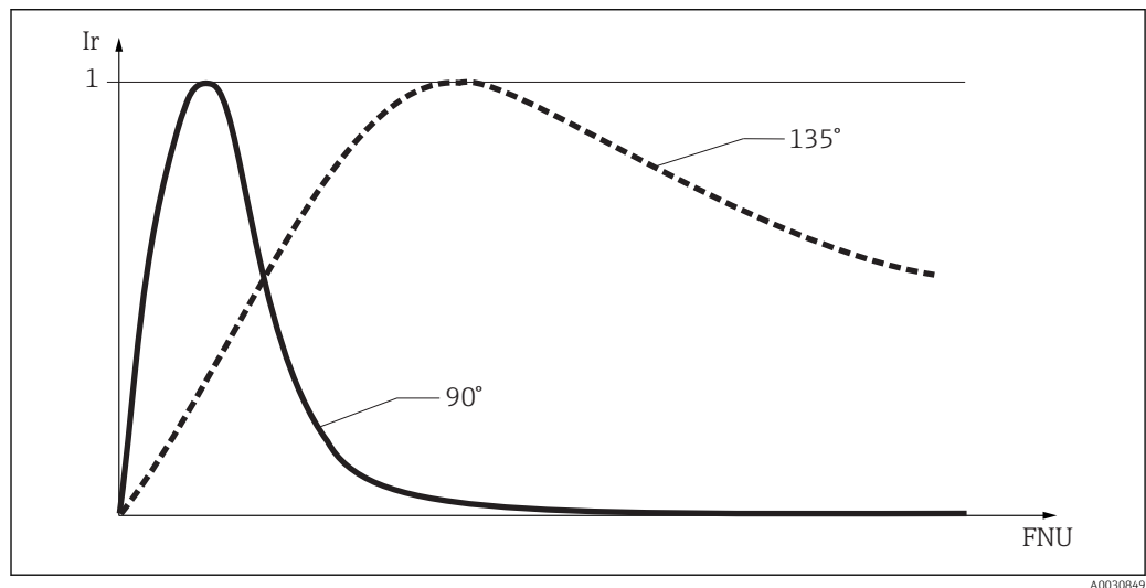
3 Распределение сигналов меняется в зависимости от содержания взвешенных частиц
