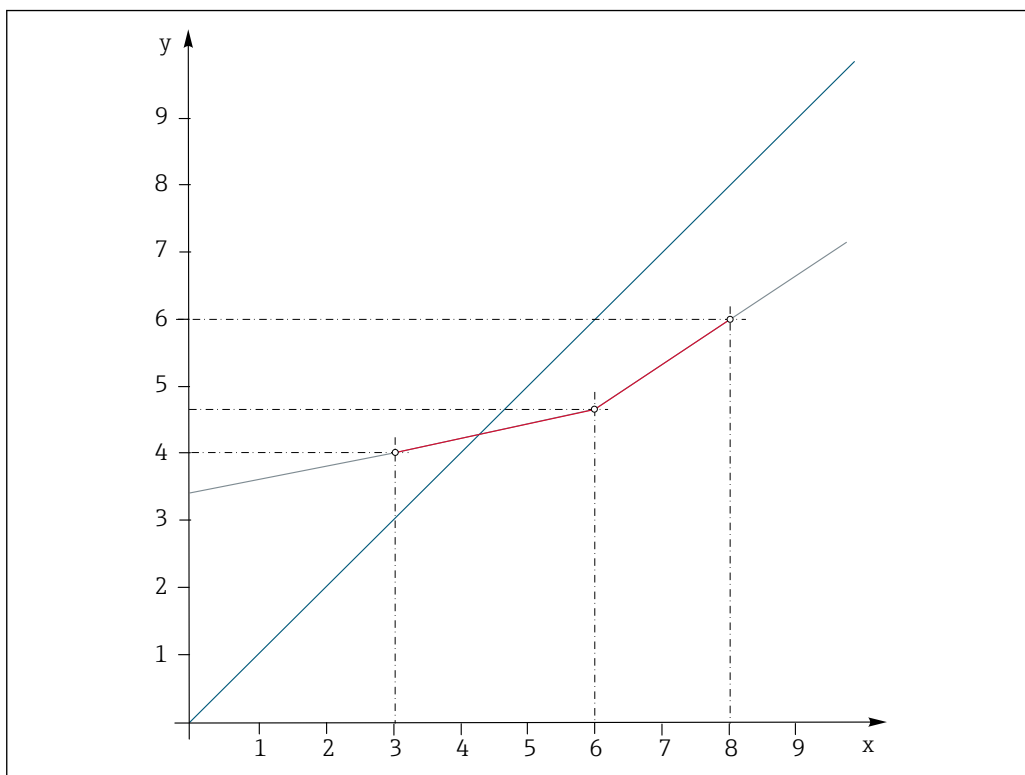
28 Принцип многоточечной калибровки (3 точки)
