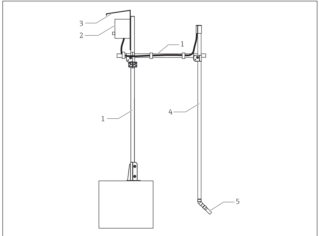
9 Измерительная система с погружной арматурой (пример)
